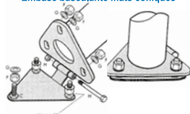
Embase basculante mats coniques
