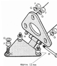
Embase basculante mats côniques
