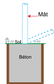
Platine Basculante
