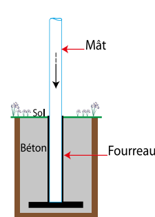
Fourreau
